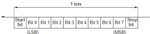
Fig. 3 Actual waveform for 1 byte
